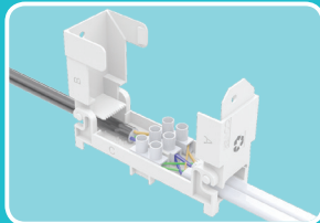
Step 3 - Insert lids
